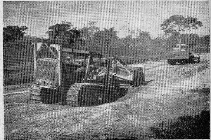
Tractor y Tounadozer equipados con trailas acarreado material selecto, de un pozo de préstamo, para formar la subbase.
