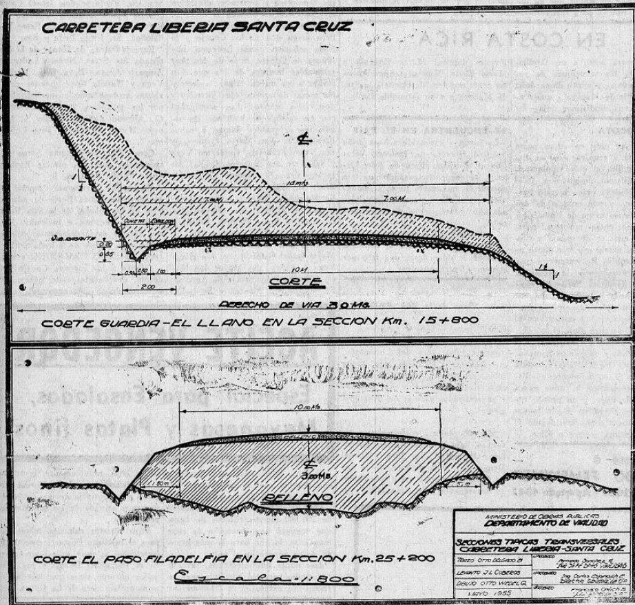
Gráfico mostrando el diseño de la Carretera Santa Cruz - Liberia
