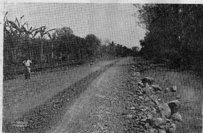
Zona derecha de préstamo y primer riego de lastre en Comunidad
